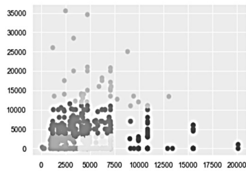
Fig. 6. EM cluster assignment, n=5
